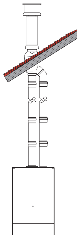
Exemple d'aspiration et évacuation au toit
